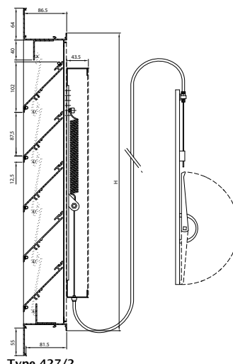
Type 427/2 Kabelbediening tot 2250 mm Minimumhoogte van het rooster 390 mm
