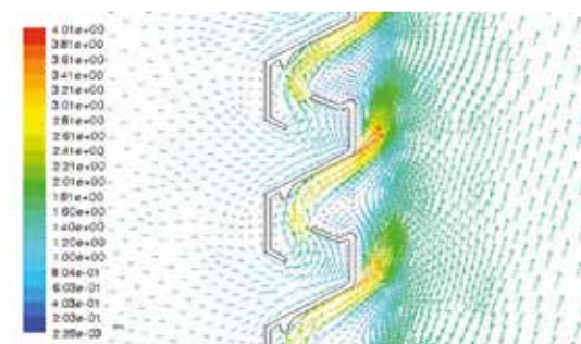
Aanzuig
