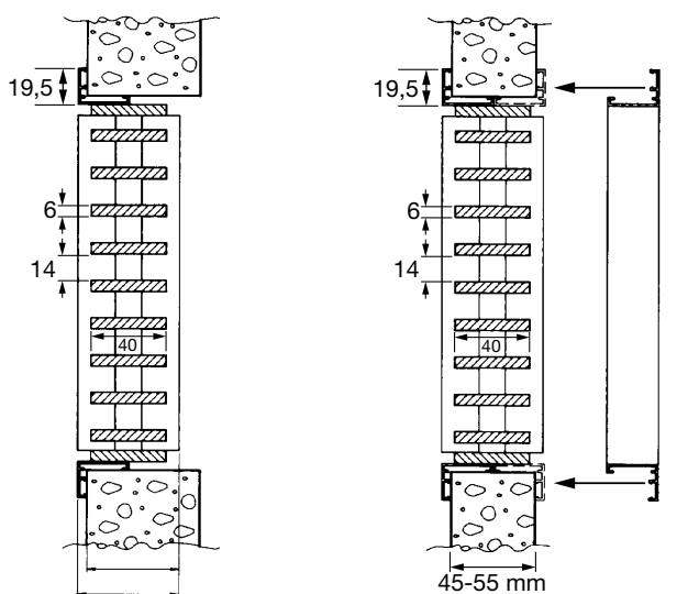
466/1 met kader
