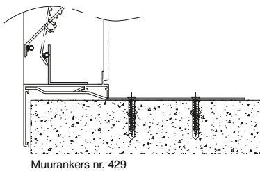
Muurankers nr. 429
